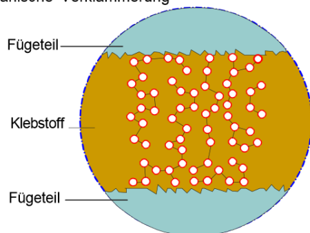
Mechanische Verklammerung
